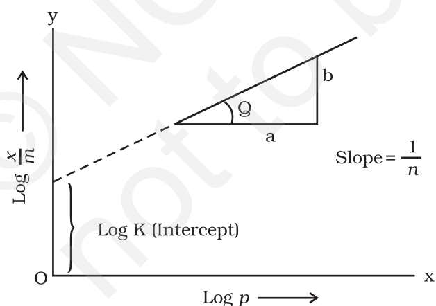
Fig. 5.2: Freundlich isotherm
